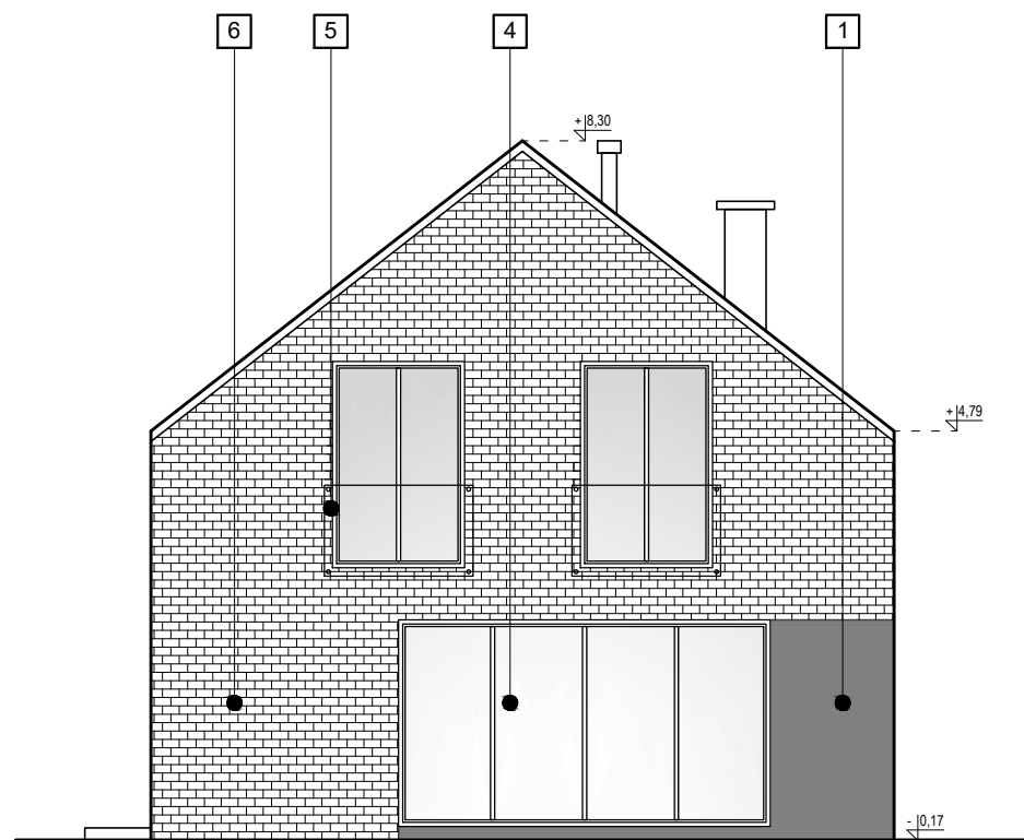
ELEWACJA POŁUDNIOWA
