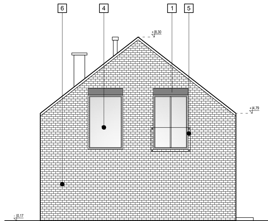
ELEWACJA PÓŁNOCNA
